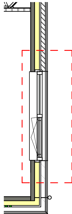
9400400 Zijgevelkozijn (circa 2.000 x 1.400 mm)
