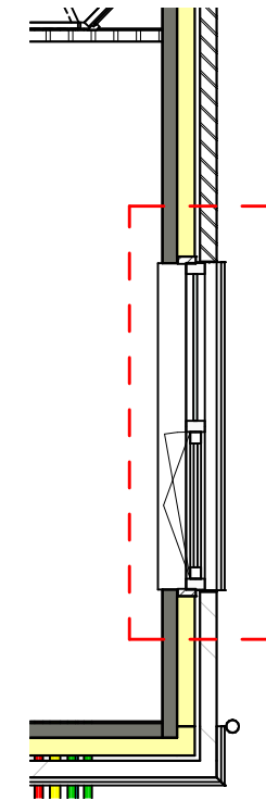
9400500 Zijgevelkozijn (circa 2.000 x 1.700 mm)
