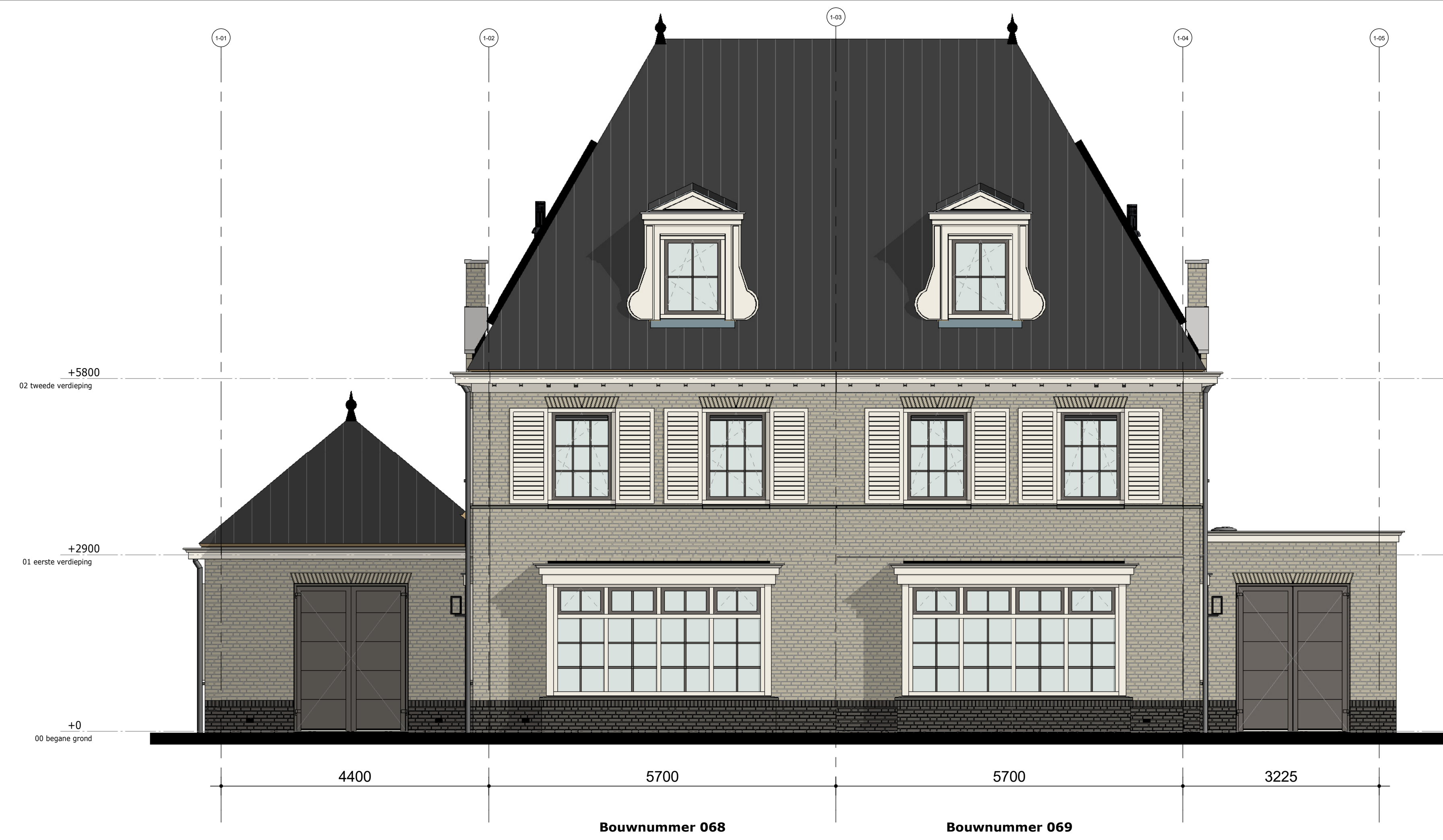
Voorgevel
