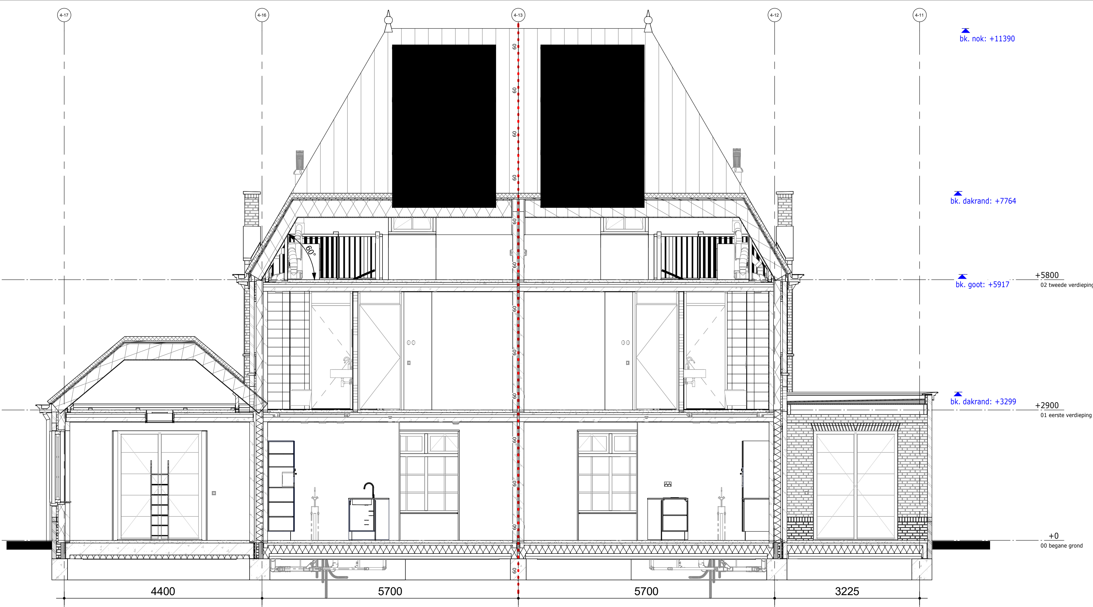
Dwarsdoorsnede
