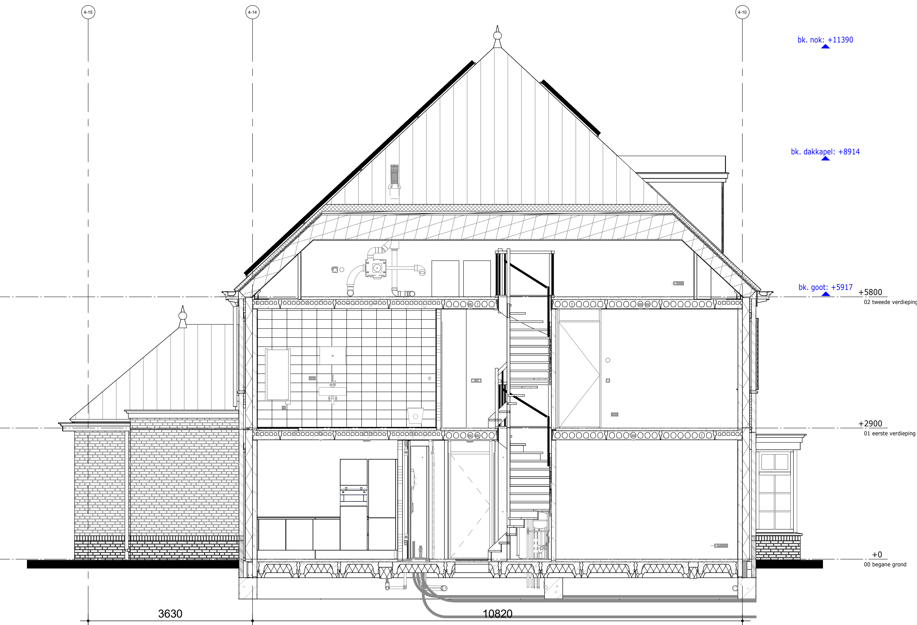
Langsdoorsnede
