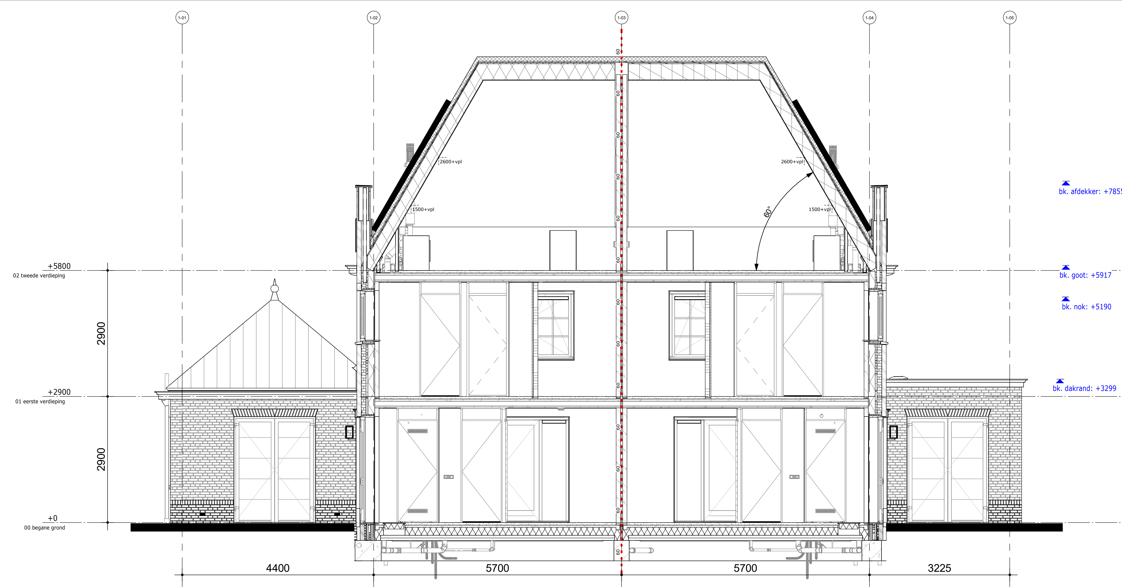
Dwarsdoorsnede
