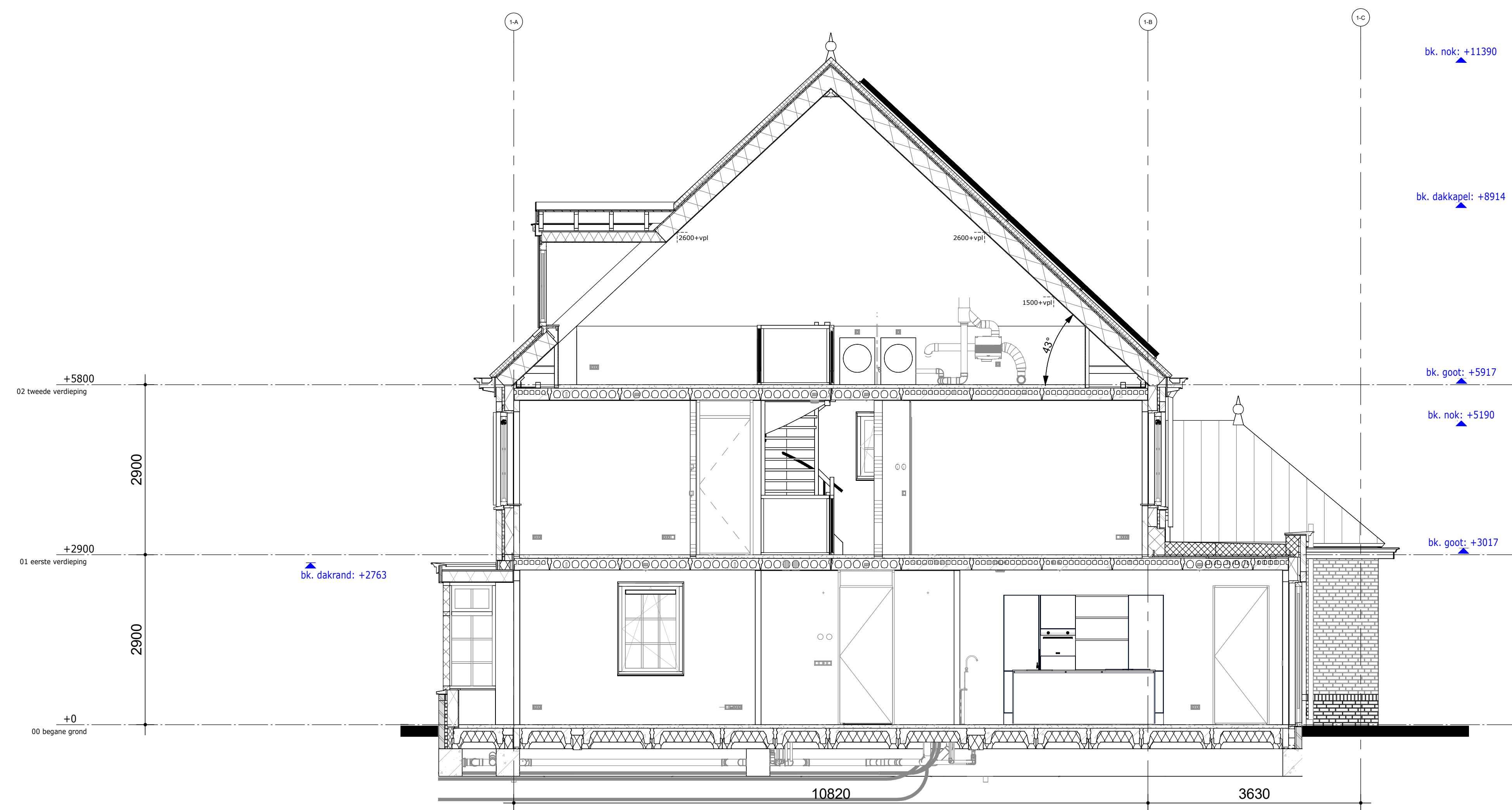
Langsdoorsnede
