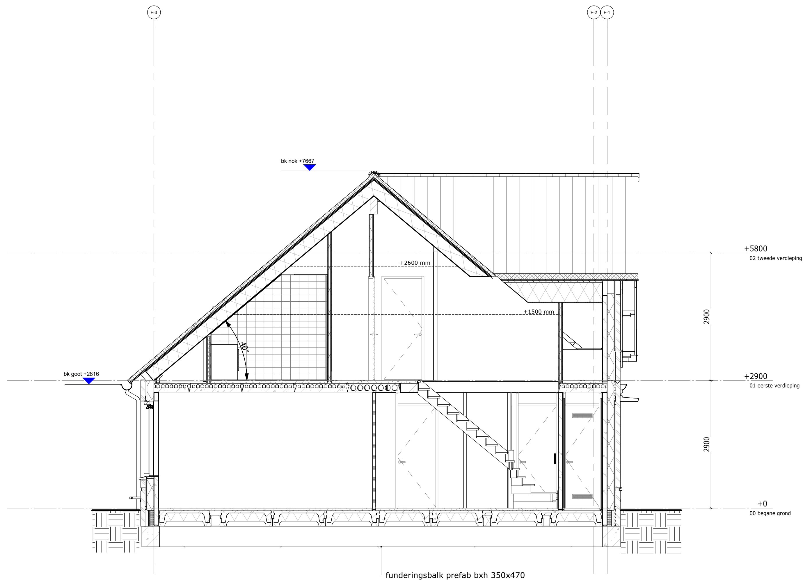
Dwarsdoorsnede
