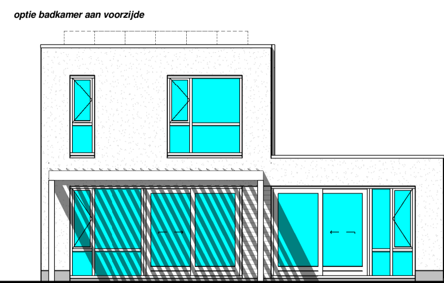
optie terrasoverkapping optie schulpui # = colorbel achtergevel opties 1 1 : 100
