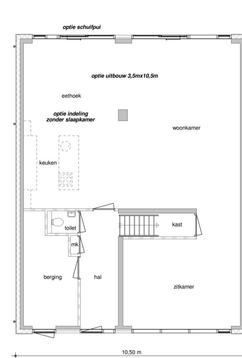
begane grond opties 5 1 : 100
