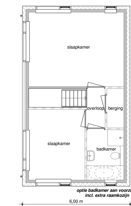
eerste verdieping opties 1 1 : 100
