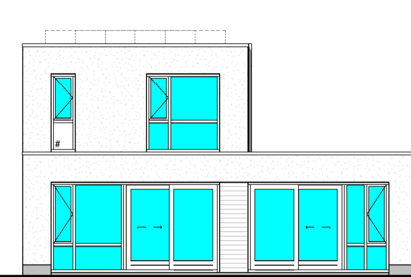
optie uitbouw 3,5mx10,5m optie schulpui # = colorbel achtergevel opties 5 1 : 100
