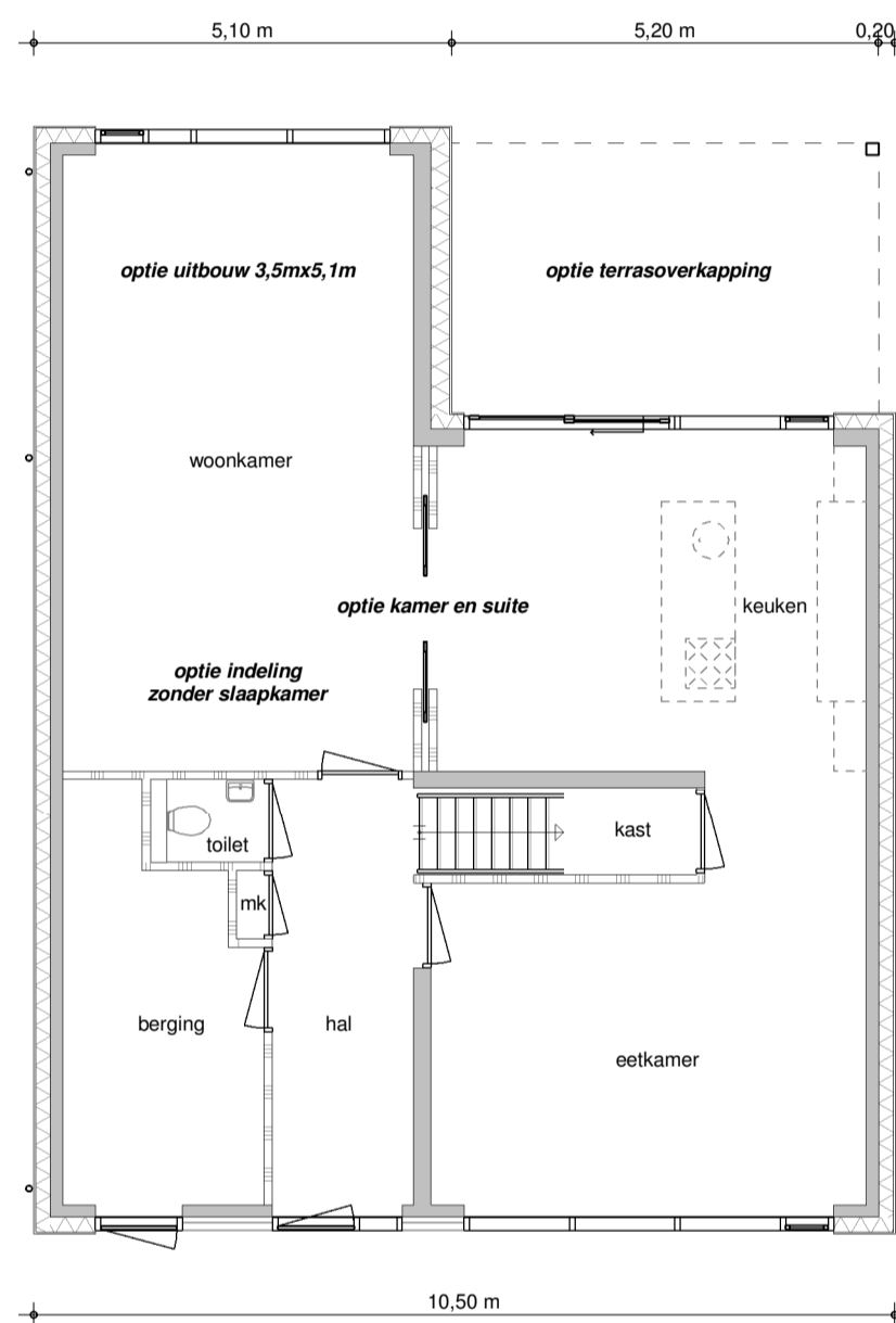
begane grond opties 3 1 : 100
