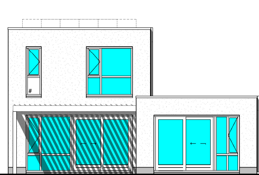
optie terrasoverkapping optie uitbouw 3,5mx5,1m optie schulpui # = colorbel achtergevel opties 2 1 : 100
