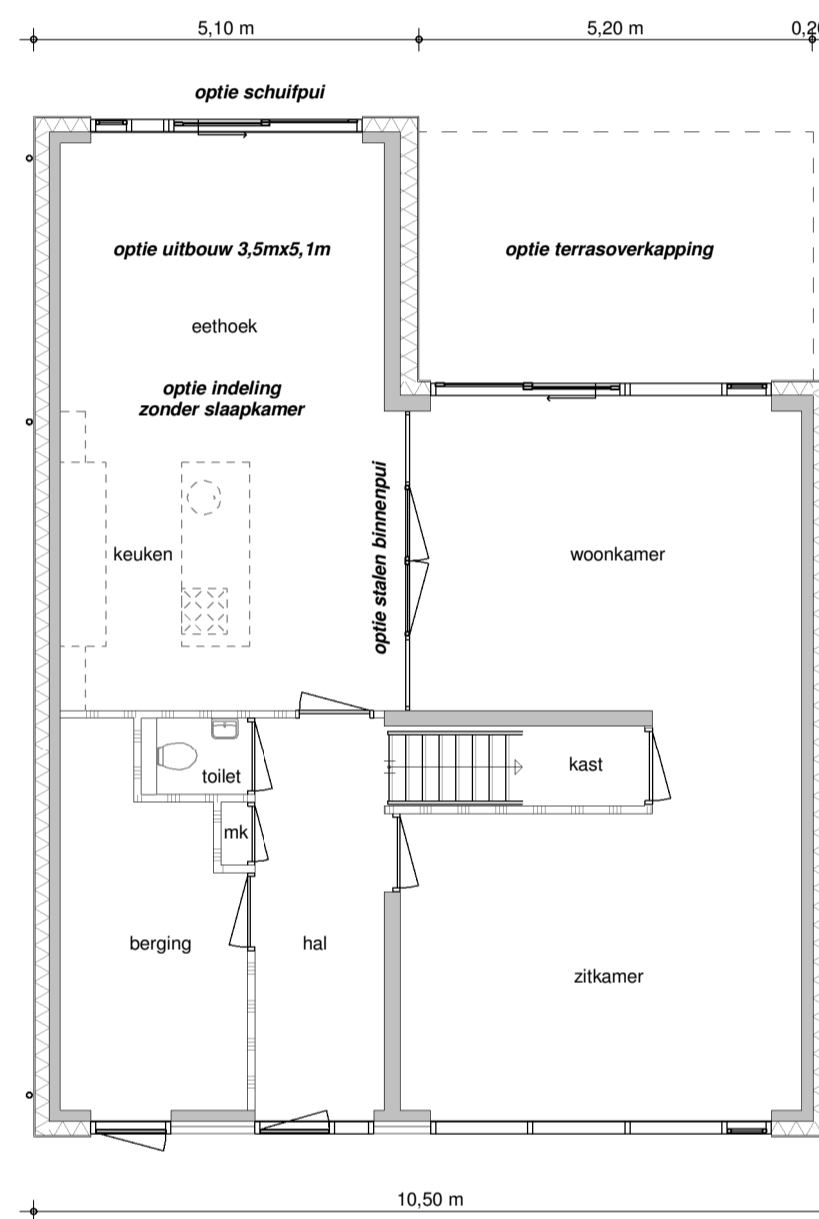
begane grond opties 4 1 : 100
