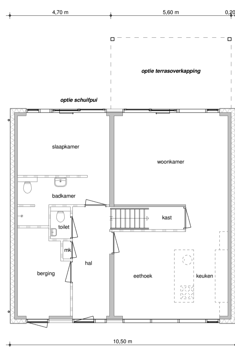
begane grond opties 1 1 : 100
