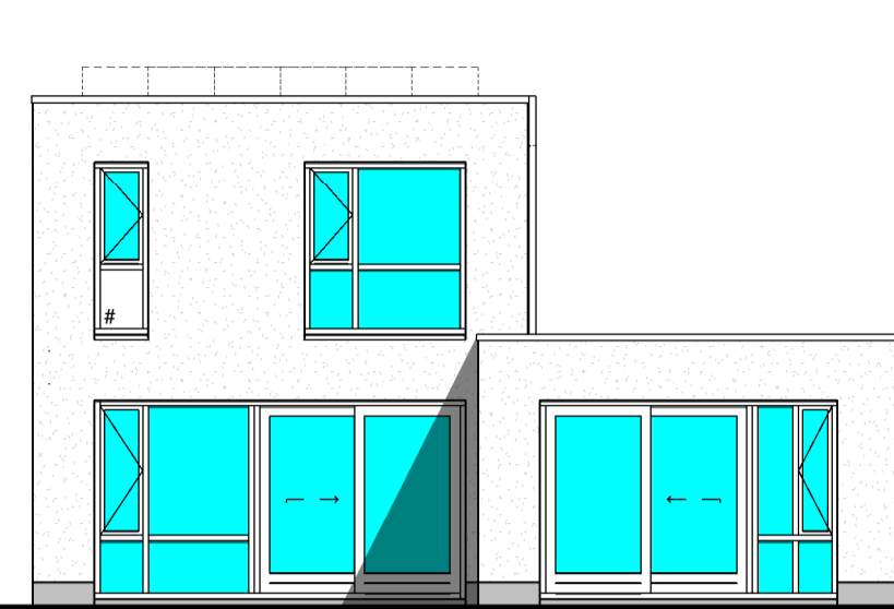
optie uitbouw 3,5mx5,1m optie schulpui # = colorbel achtergevel opties 4 1 : 100
