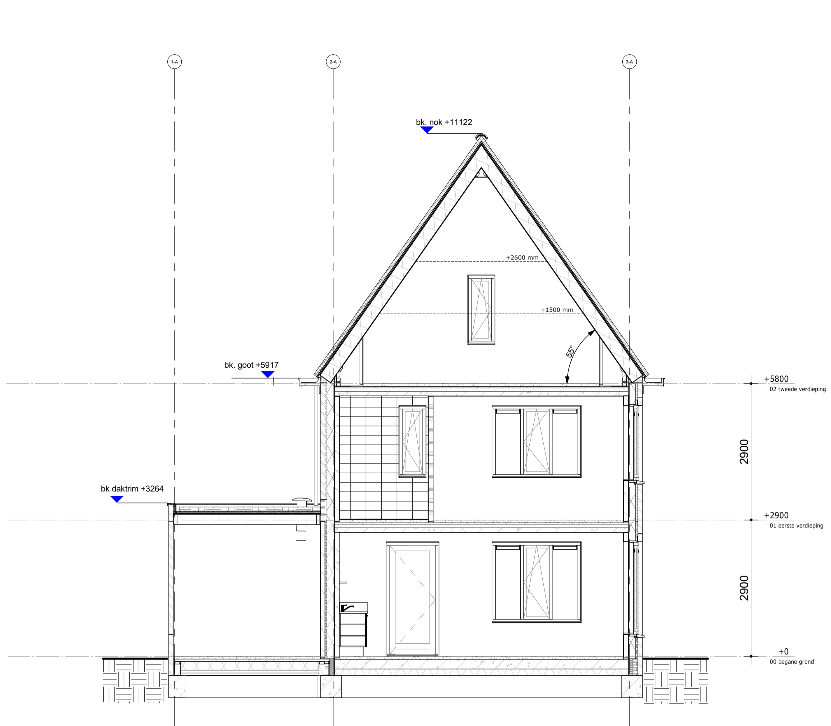
Dwarsdoorsnede
