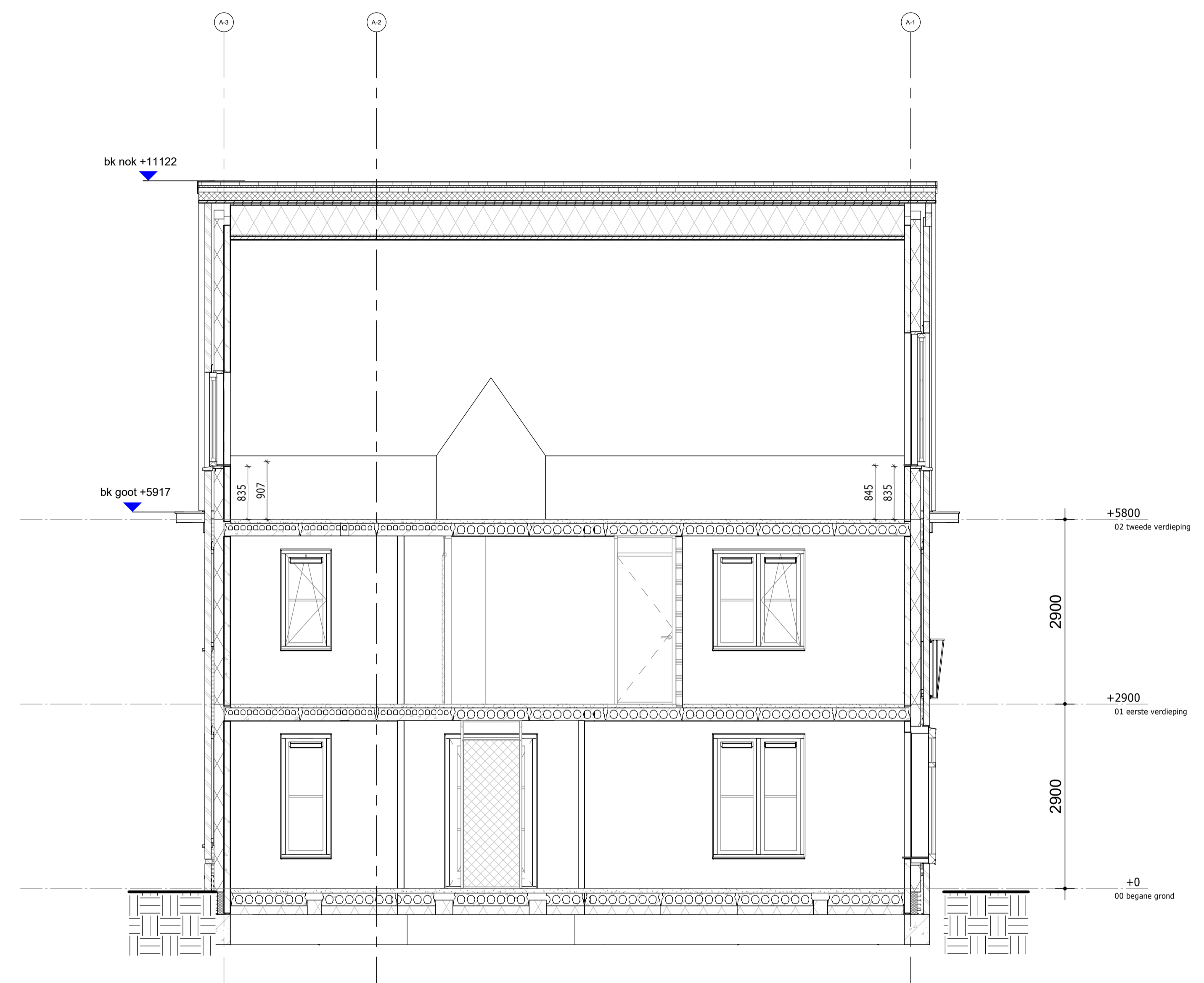
Langsdoorsnede
