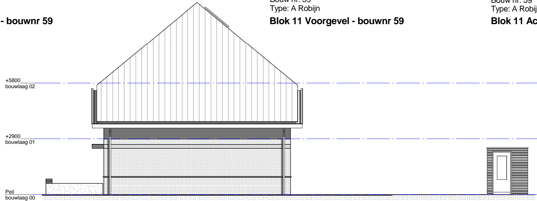
Rechter zijgevel
