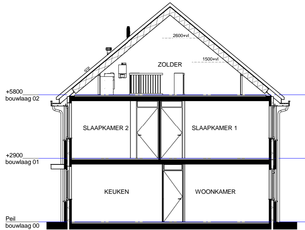
Doorsnede - bouwnr 59
