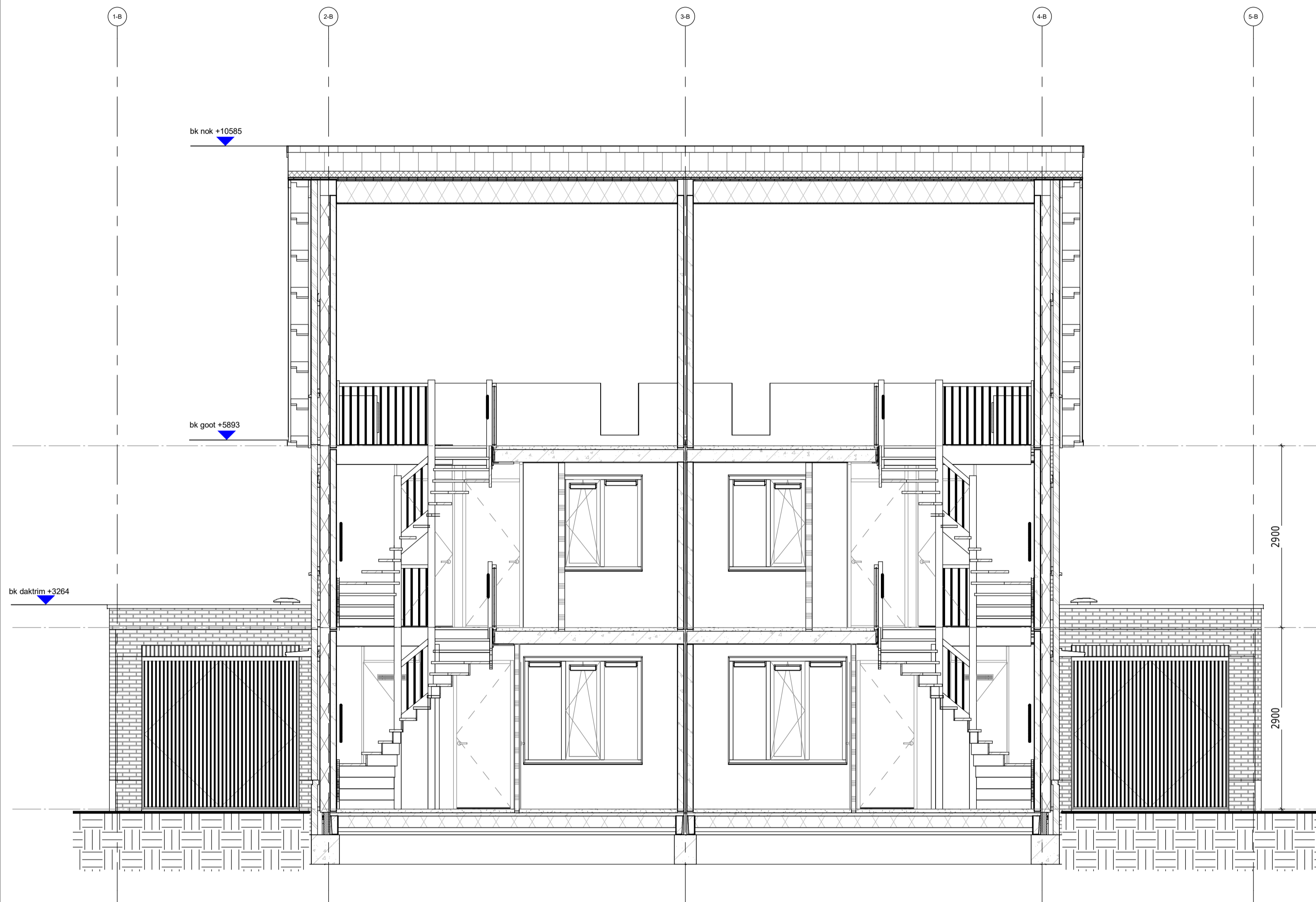
Langsdoorsnede
