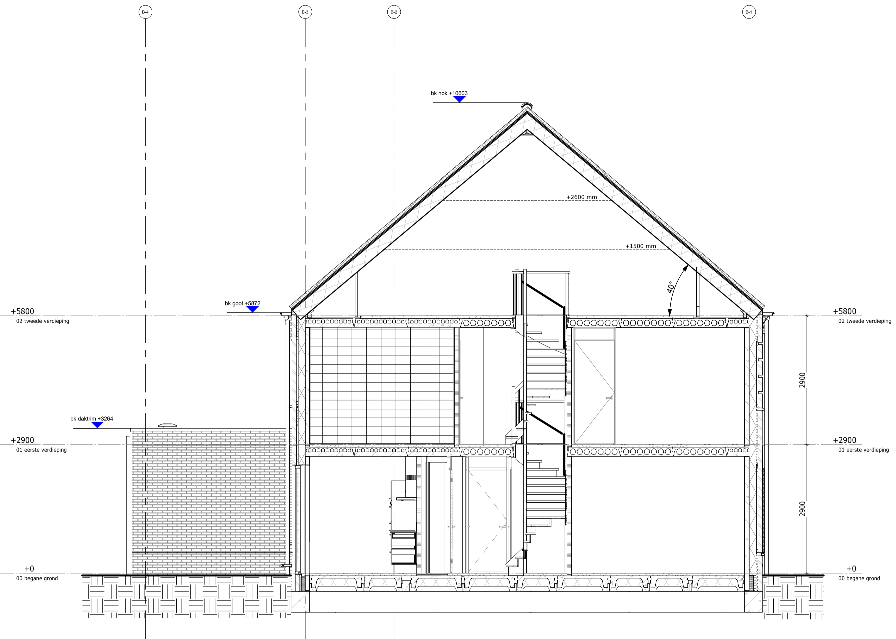
Dwarsdoorsnede
