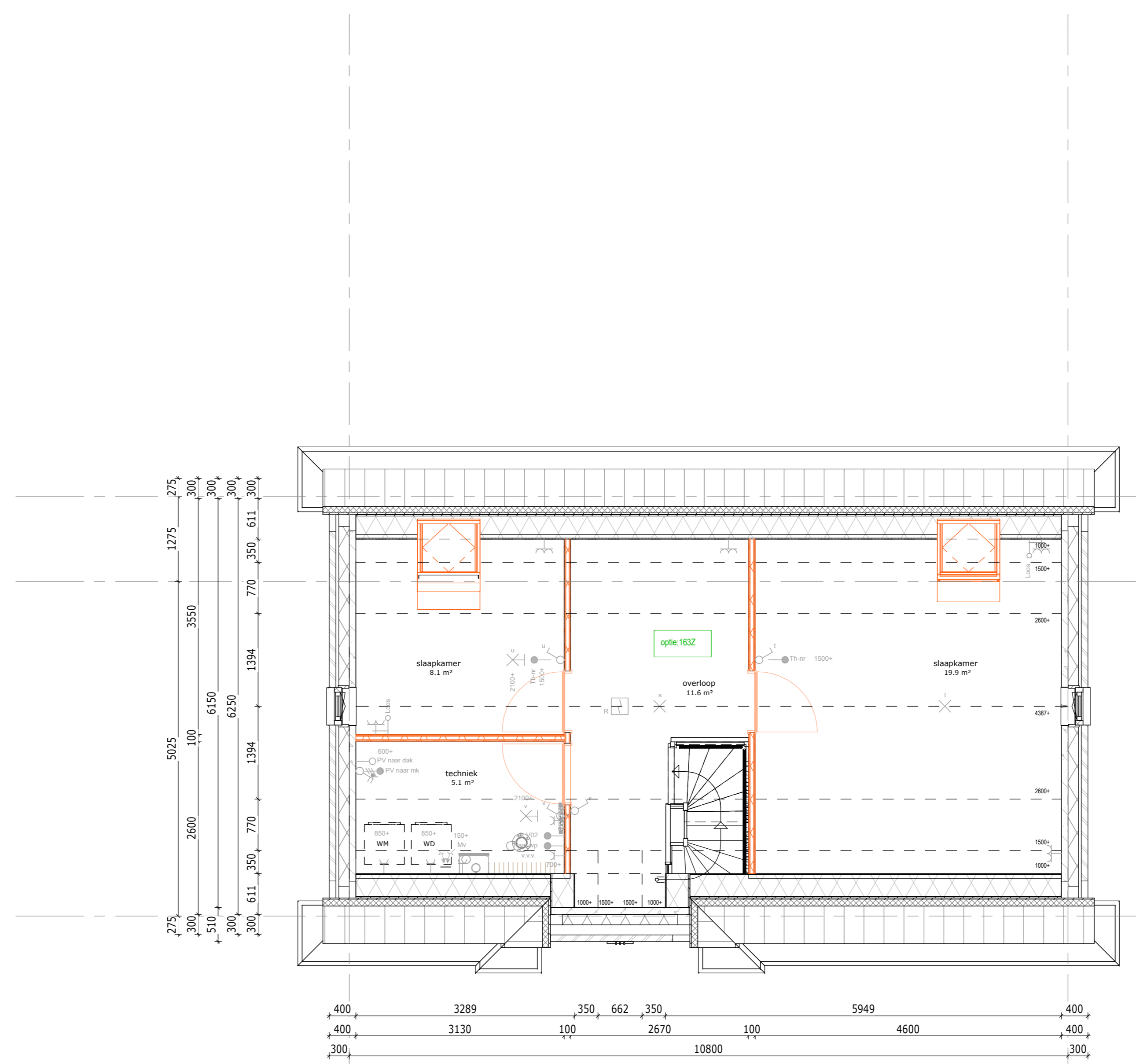
102 Zolderbelting met 2 slaapkamers en overloop
