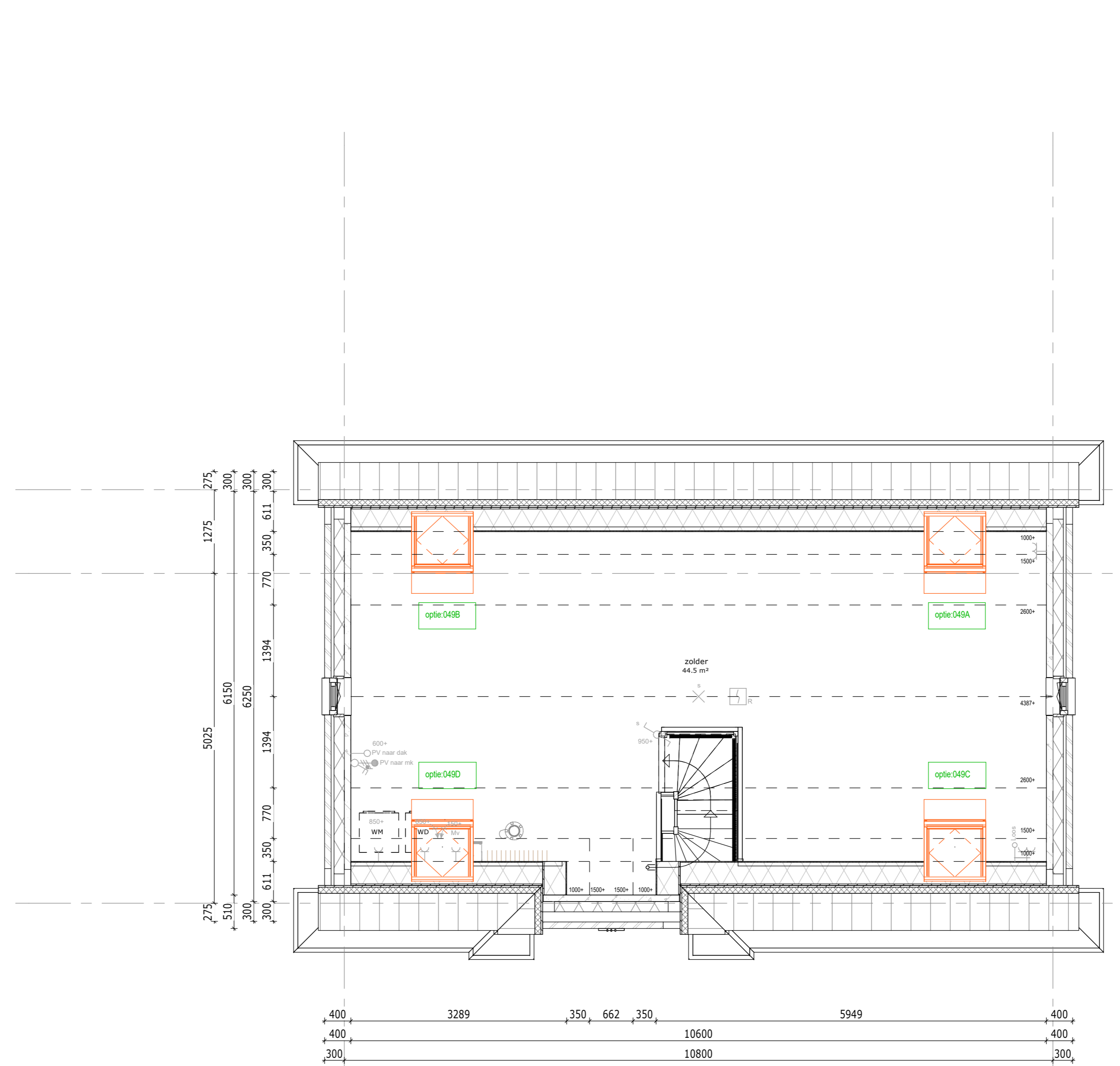
04B Dakkapel op achtergevel, breedte 2500 mm
