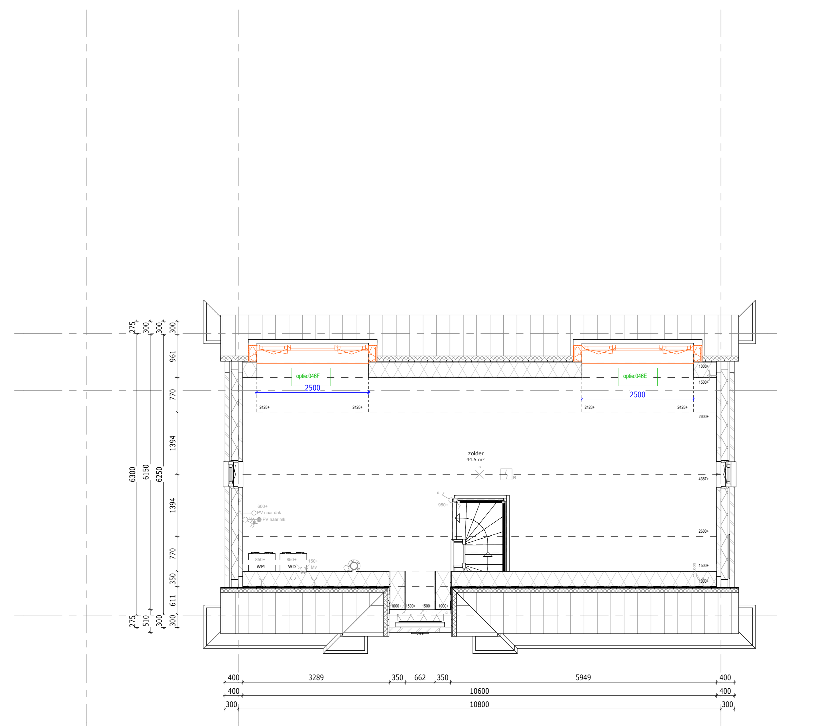
04A Dakkapel op achtergevel, breedte 2500 mm
