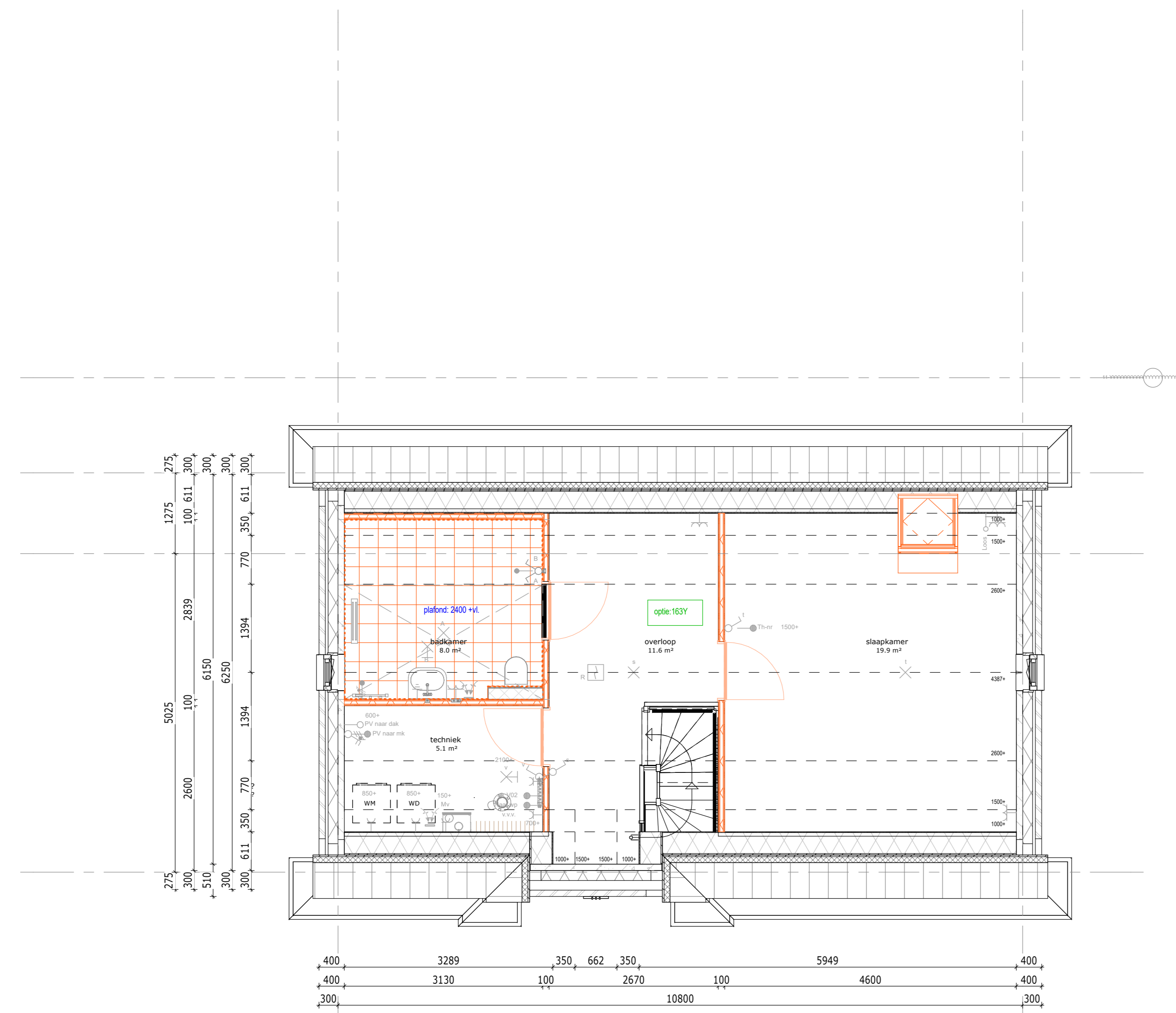
101 Zolderbelting met badkamer, slaapkamer, berggarage en techn. ruimte
